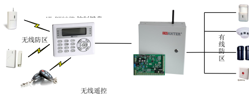
GLOBAL NT2XXW 无线扩展结构示意图
