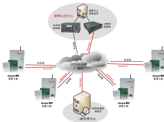
电话线/Internet 网络报警联网应用方案
