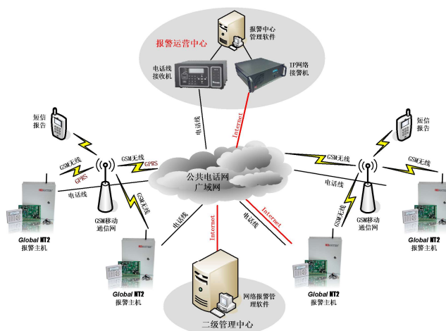
电话线数据/GPRS 网络报警联网方案
